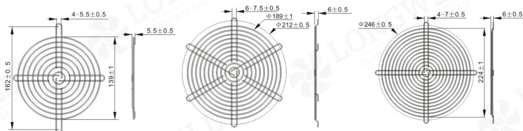
Model : LW172 Suitable for fan : LW17023/1725/17255
