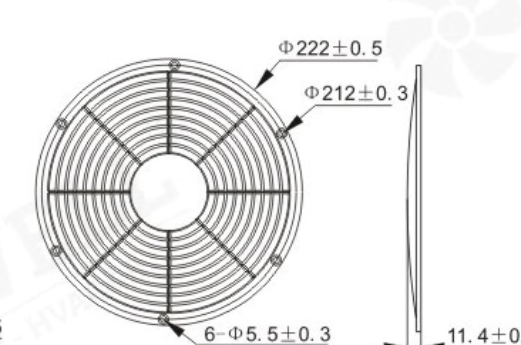
Model : LW822B Suitable for fan : LW2206/2208
