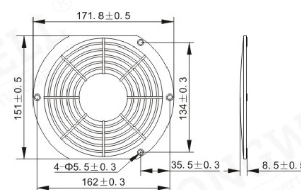
Model : LW817B Suitable for fan : LW1725/17255
