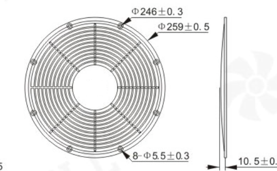
Model : LW825B Suitable for fan : LW2509
